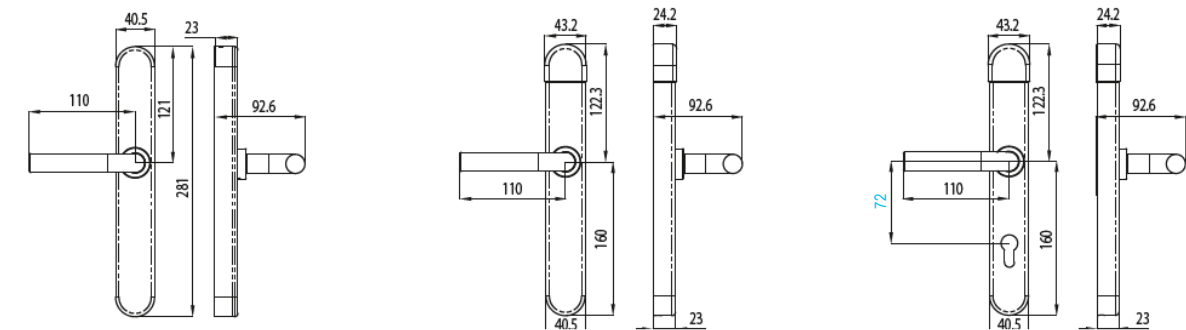
Internal Escutcheon UOC BLE L1S/L2V
