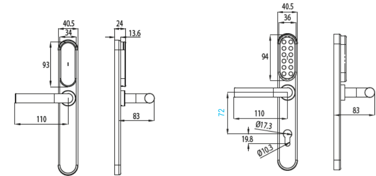
External Escutcheon L1S
